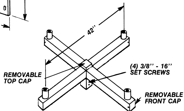
IMPSSB-4-90°
